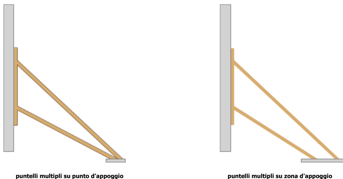
puntelli multipli su punto d'appoggio
